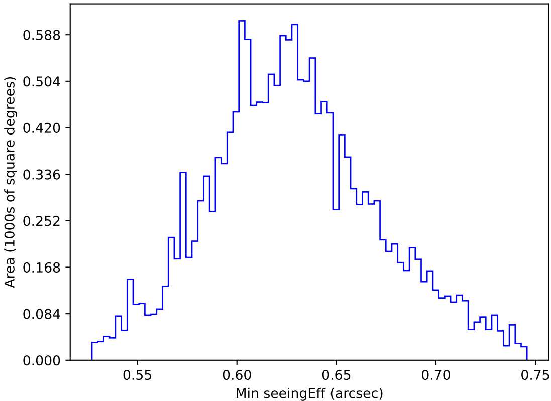
extra_ss_neo7_v3.4_10yrs WFD y band: Min seeingEff
