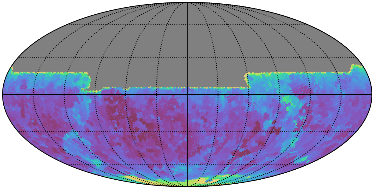
extra_ss_neo7_v3.4_10yrs All sky y band: Min seeingEff
