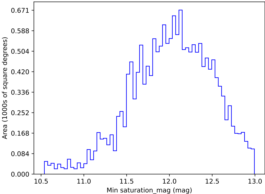
extra_ss_neo7_v3.4_10yrs WFD z band: Min saturation_mag
