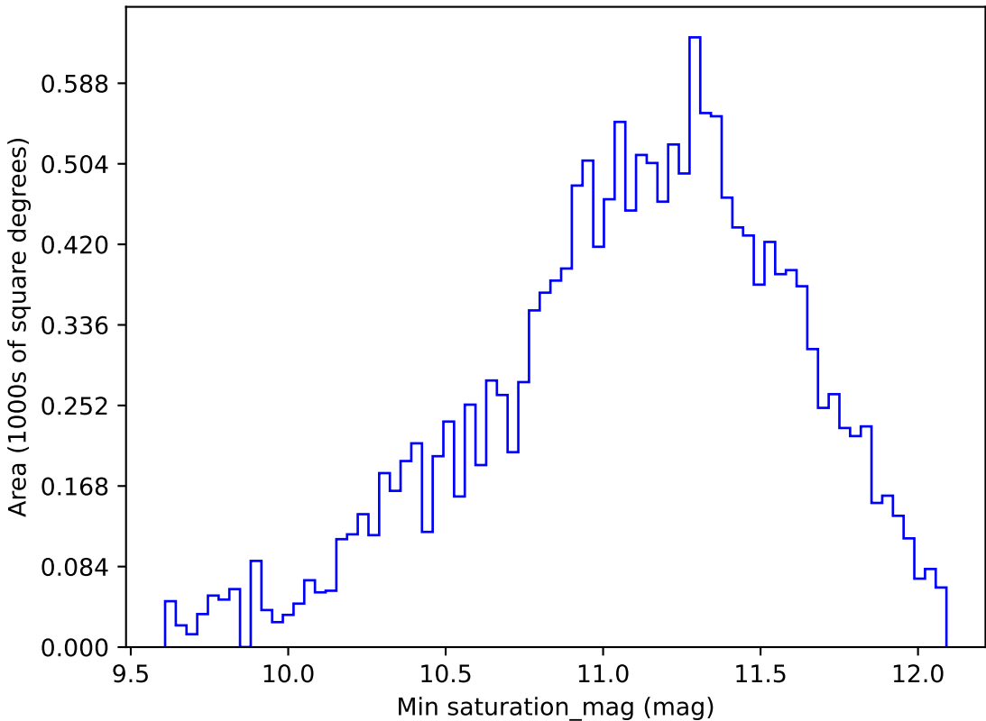
extra_ss_neo7_v3.4_10yrs WFD y band: Min saturation_mag
