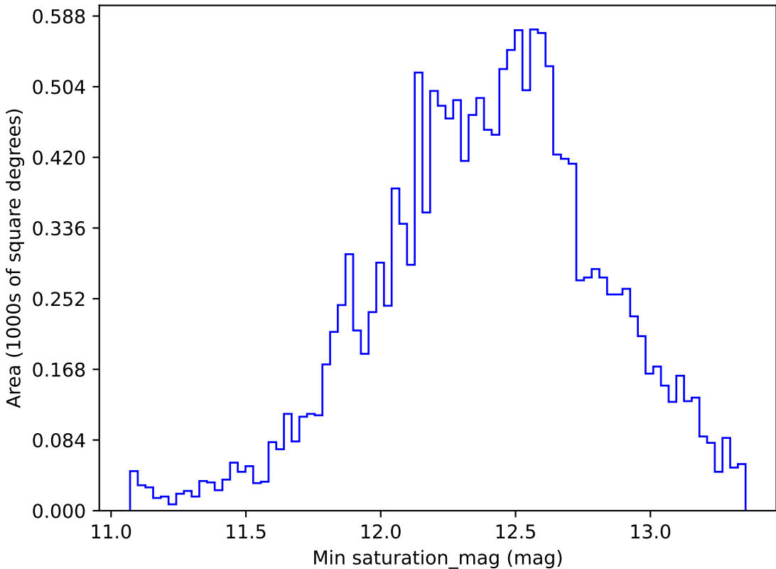
extra_ss_neo7_v3.4_10yrs WFD i band: Min saturation_mag
