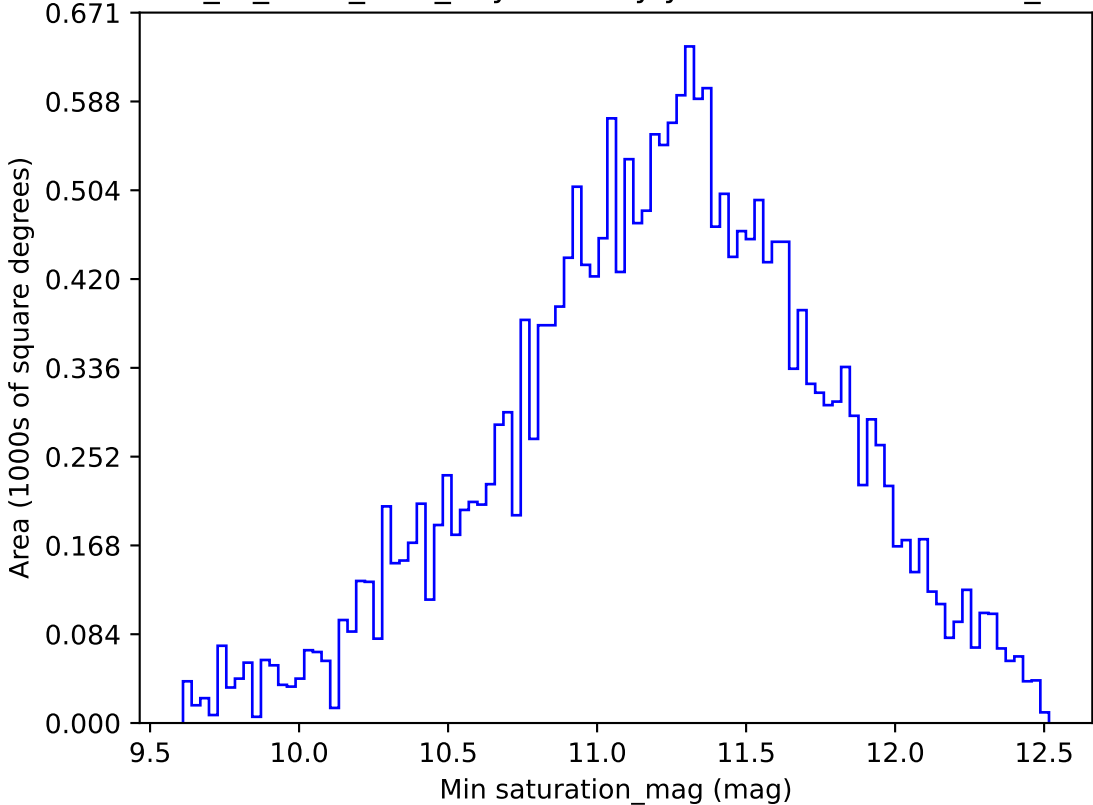
extra_ss_neo7_v3.4_10yrs All sky y band: Min saturation_mag
