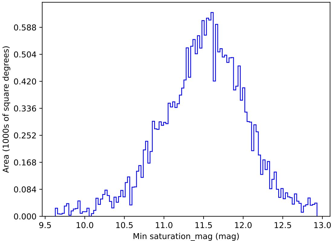
extra_ss_neo7_v3.4_10yrs All sky u band: Min saturation_mag
