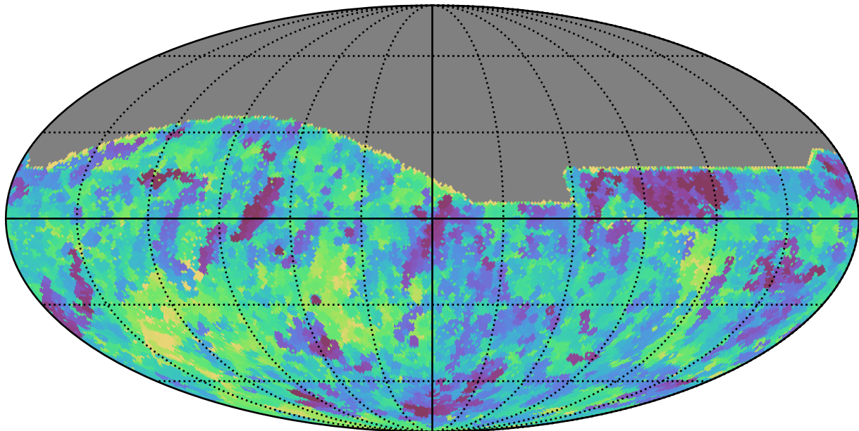
extra_ss_neo7_v3.4_10yrs All sky r band: Min saturation_mag
