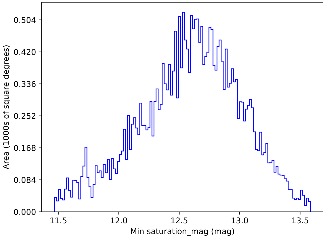
extra_ss_neo7_v3.4_10yrs All sky r band: Min saturation_mag
