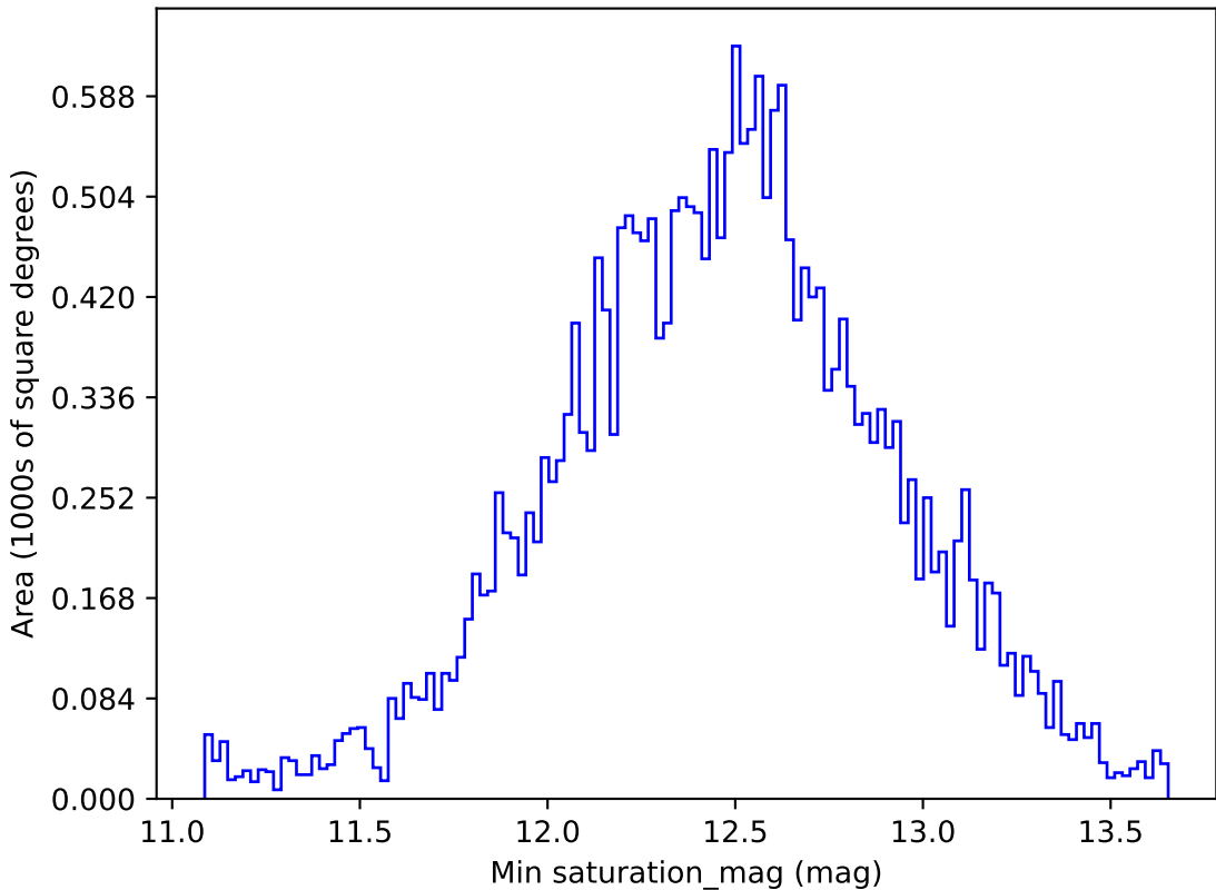
extra_ss_neo7_v3.4_10yrs All sky i band: Min saturation_mag
