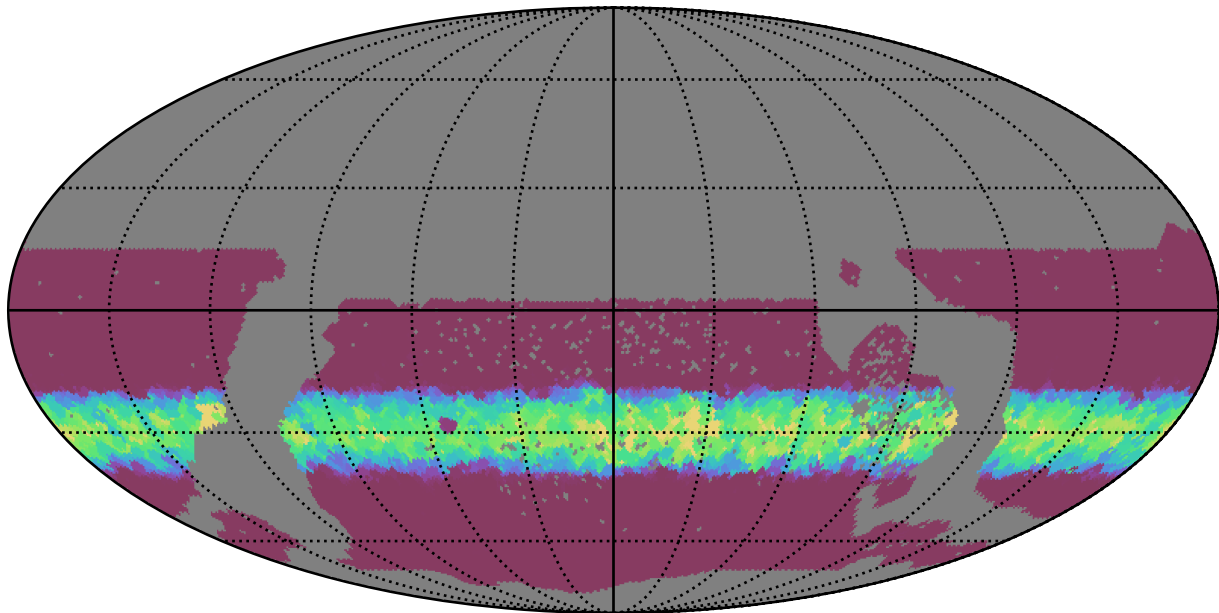
extra_ss_neo7_v3.4_10yrs WFD z band: Min normairmass
