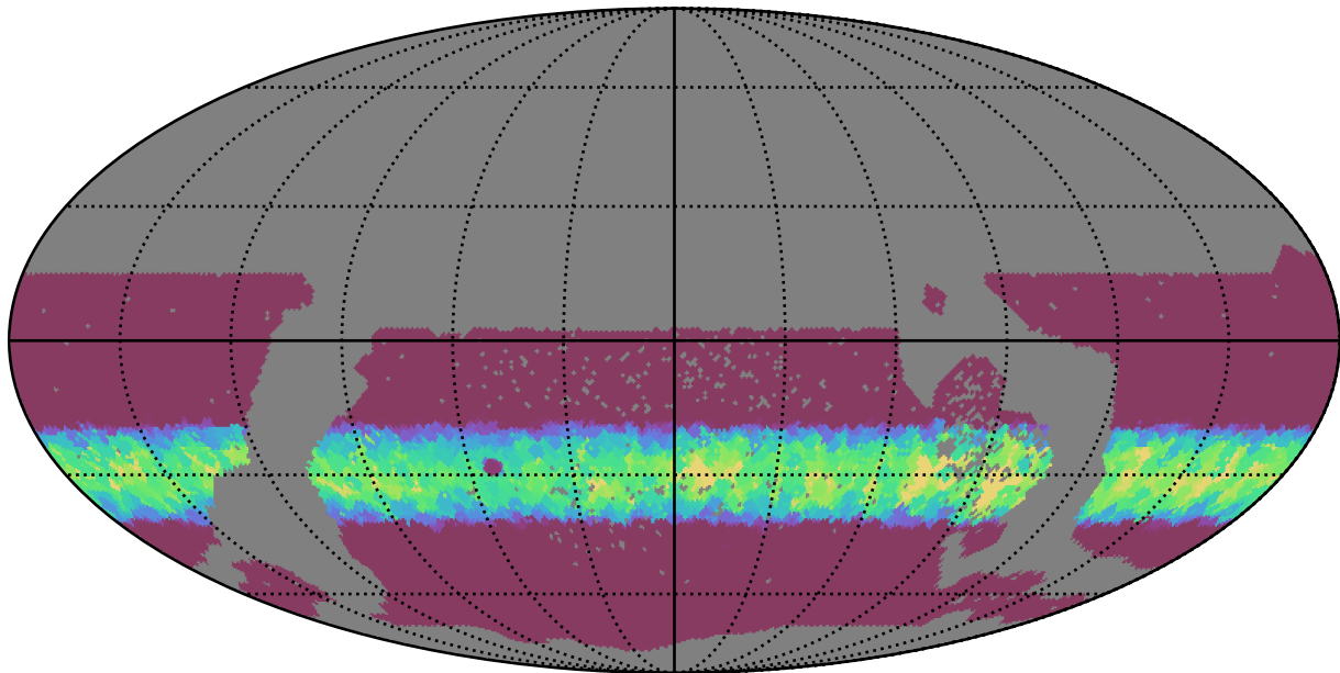
extra_ss_neo7_v3.4_10yrs WFD y band: Min normairmass
