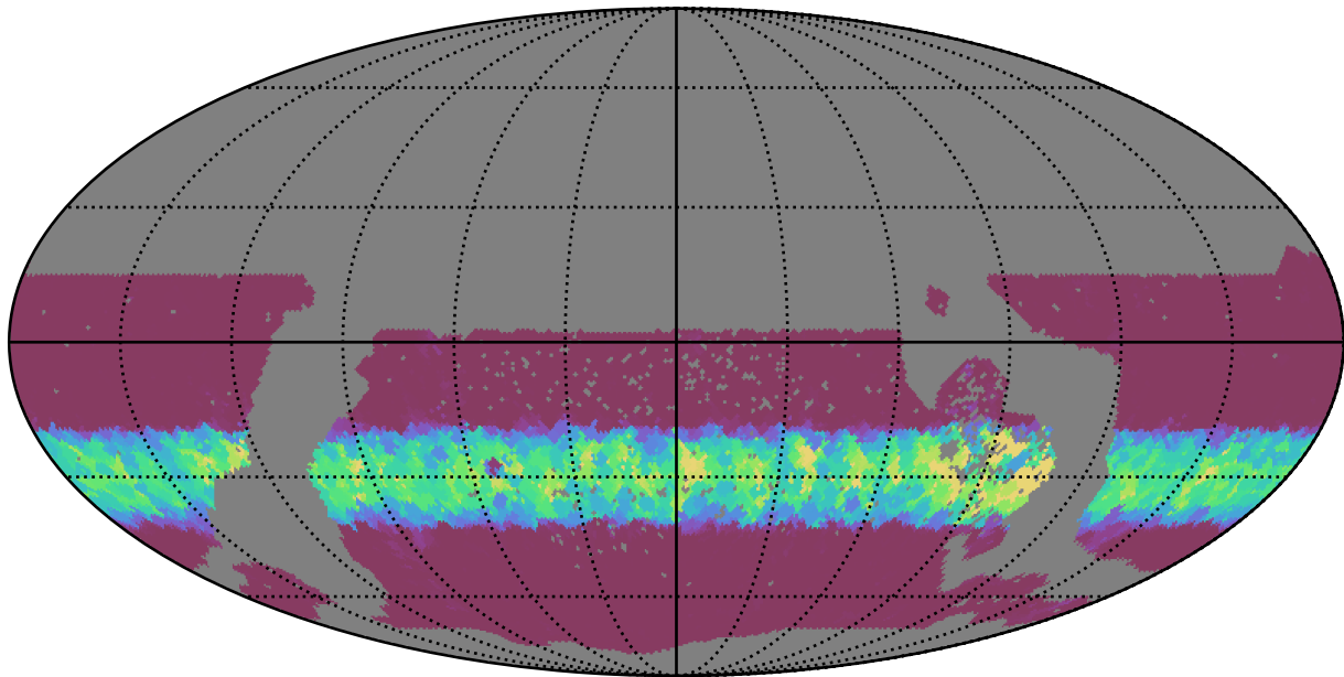
extra_ss_neo7_v3.4_10yrs WFD u band: Min normairmass
