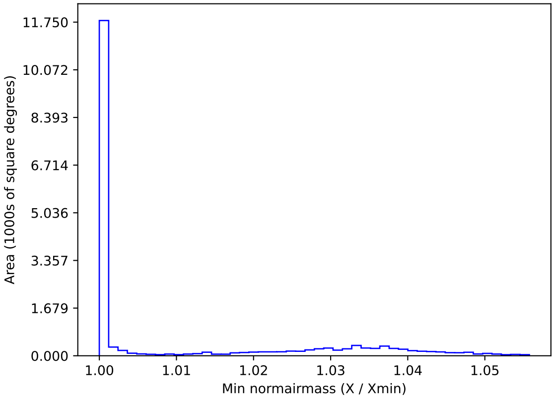
extra_ss_neo7_v3.4_10yrs WFD u band: Min normairmass
