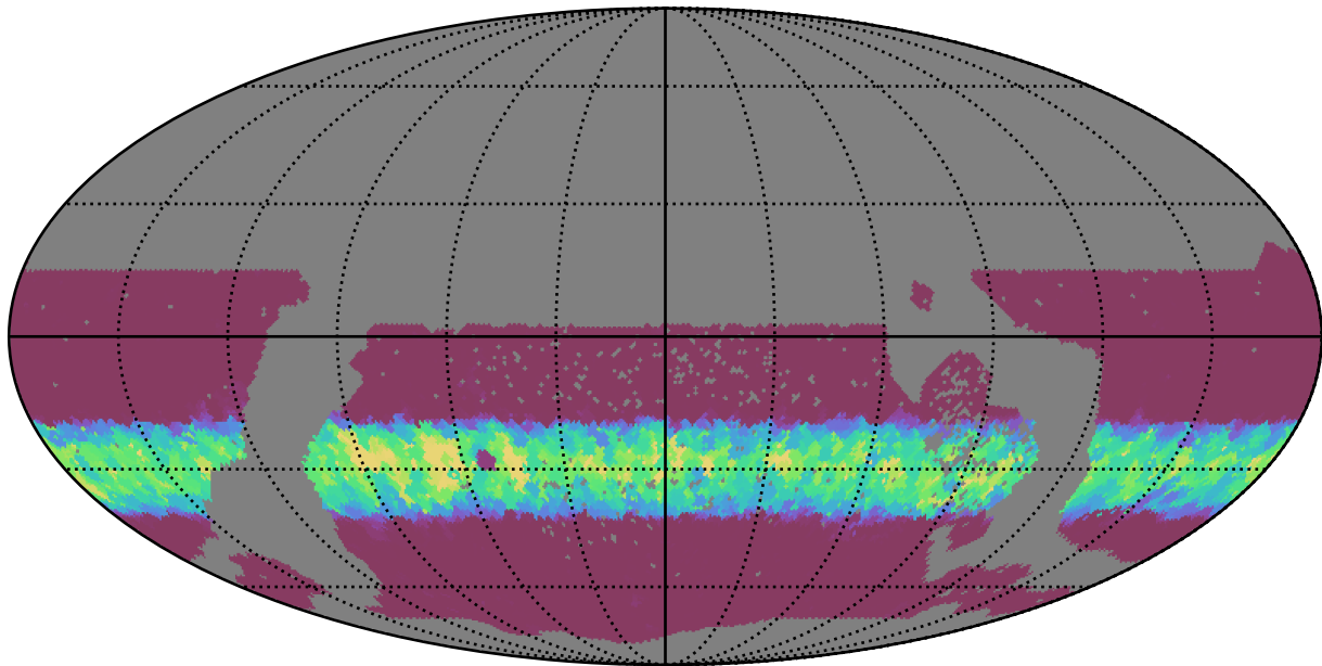
extra_ss_neo7_v3.4_10yrs WFD g band: Min normairmass
