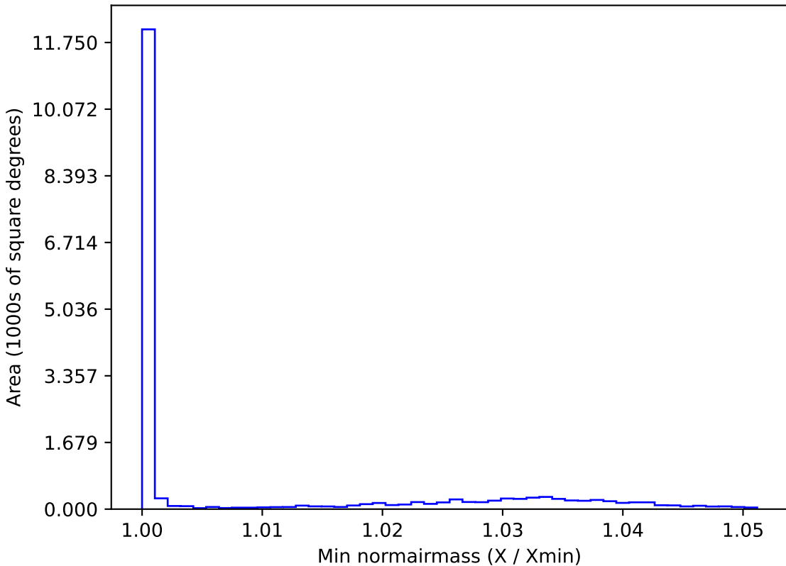
extra_ss_neo7_v3.4_10yrs WFD g band: Min normairmass
