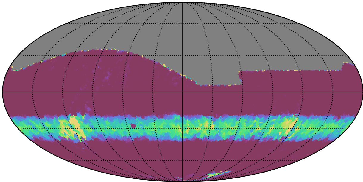
extra_ss_neo7_v3.4_10yrs All sky z band: Min normairmass
