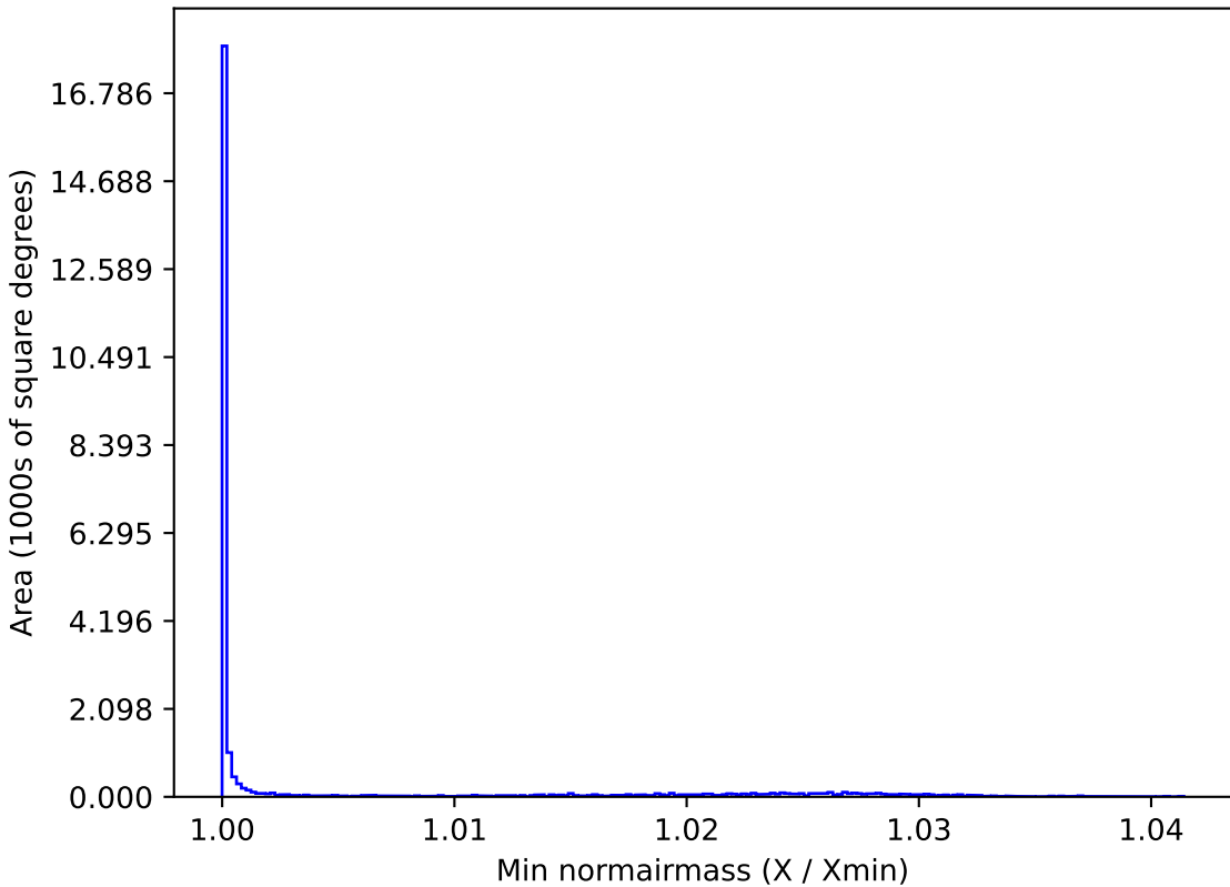
extra_ss_neo7_v3.4_10yrs All sky z band: Min normairmass
