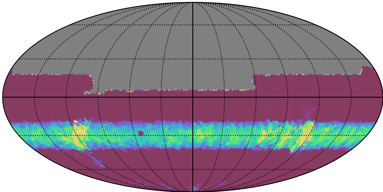
extra_ss_neo7_v3.4_10yrs All sky y band: Min normairmass
