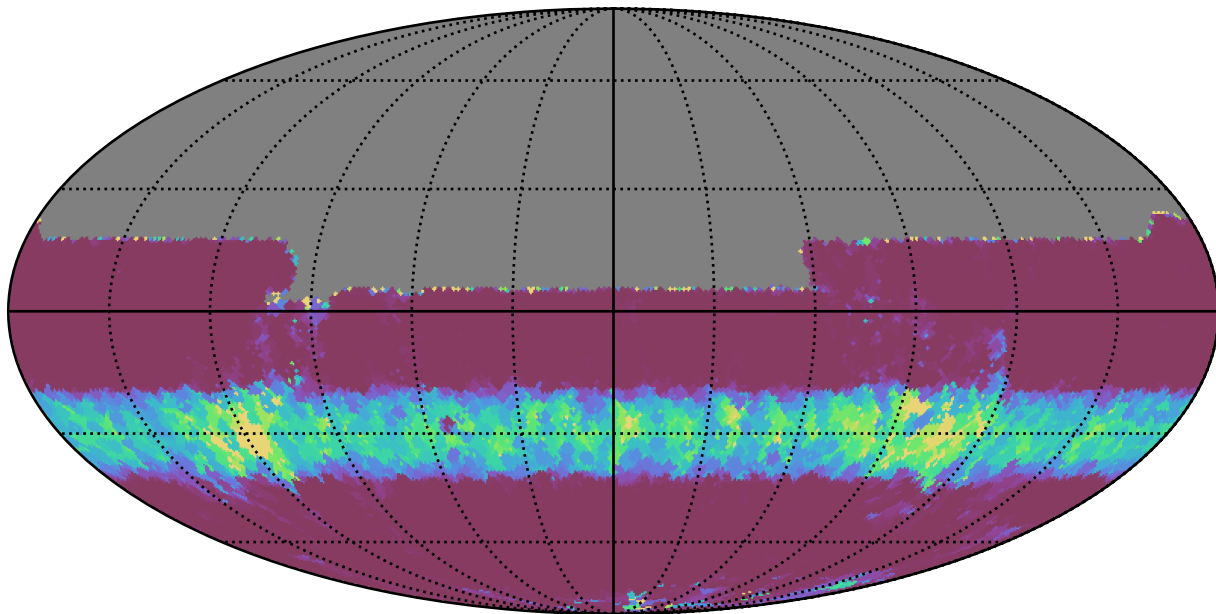
extra_ss_neo7_v3.4_10yrs All sky u band: Min normairmass
