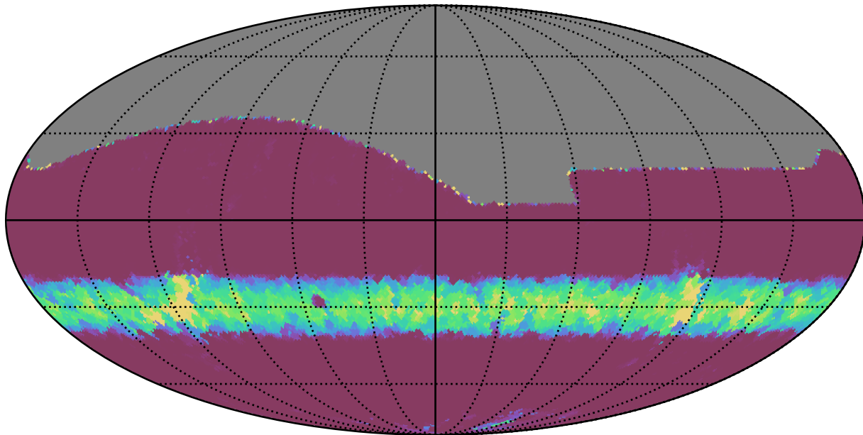
extra_ss_neo7_v3.4_10yrs All sky i band: Min normairmass
