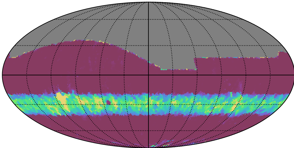
extra_ss_neo7_v3.4_10yrs All sky g band: Min normairmass
