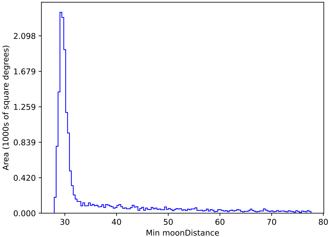
extra_ss_neo7_v3.4_10yrs WFD z band: Min moonDistance
