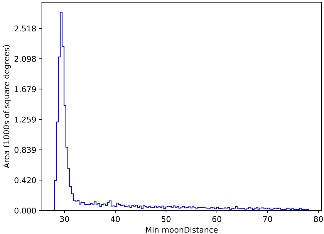
extra_ss_neo7_v3.4_10yrs WFD y band: Min moonDistance
