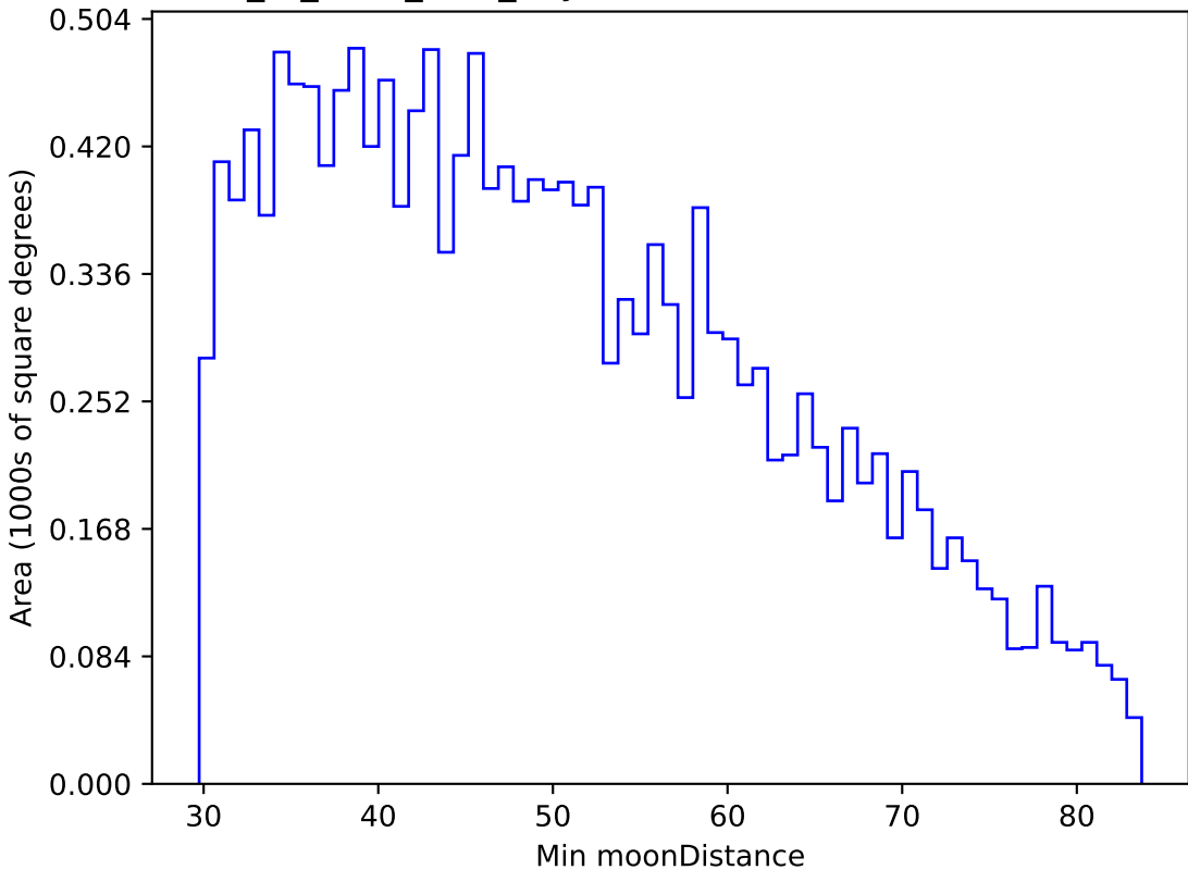
extra_ss_neo7_v3.4_10yrs WFD u band: Min moonDistance
