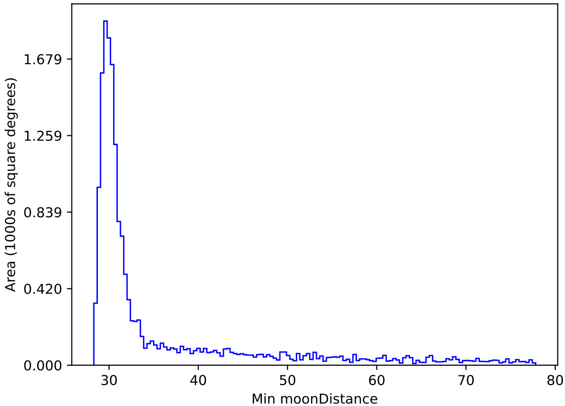
extra_ss_neo7_v3.4_10yrs WFD i band: Min moonDistance
