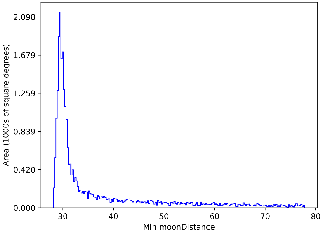
extra_ss_neo7_v3.4_10yrs All sky z band: Min moonDistance
