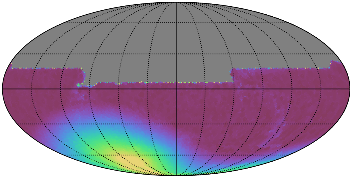
extra_ss_neo7_v3.4_10yrs All sky y band: Min moonDistance
