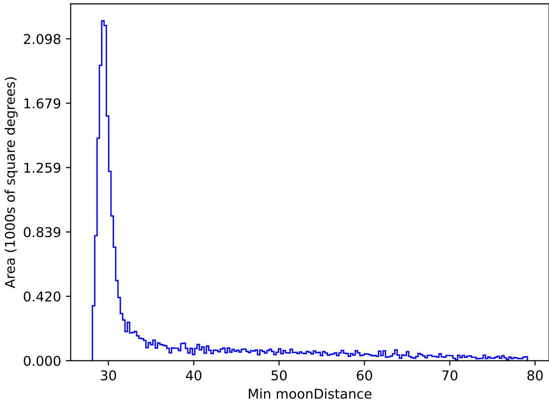
extra_ss_neo7_v3.4_10yrs All sky y band: Min moonDistance
