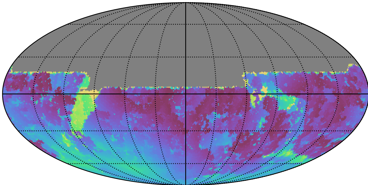
extra_ss_neo7_v3.4_10yrs All sky u band: Min moonDistance
