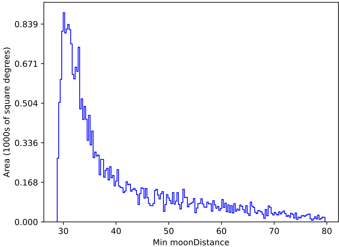
extra_ss_neo7_v3.4_10yrs All sky r band: Min moonDistance
