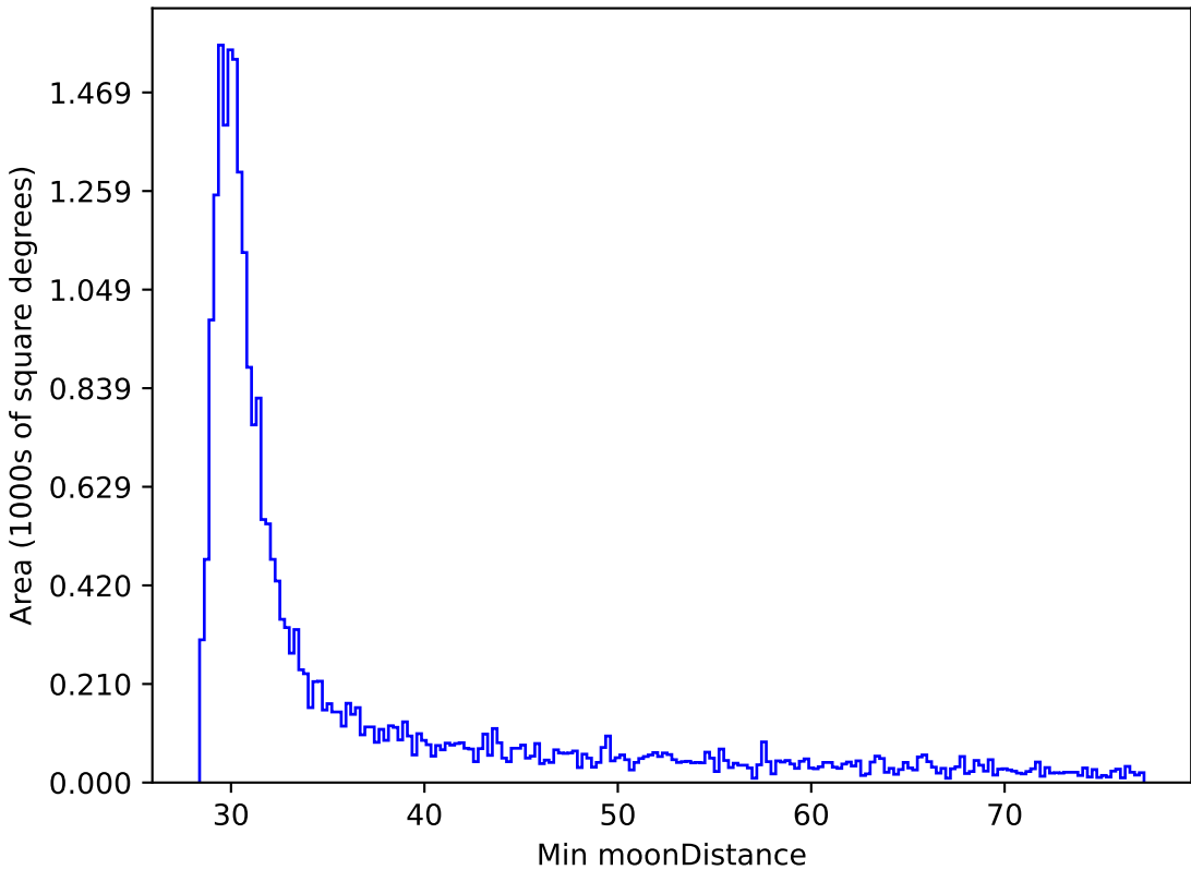
extra_ss_neo7_v3.4_10yrs All sky i band: Min moonDistance
