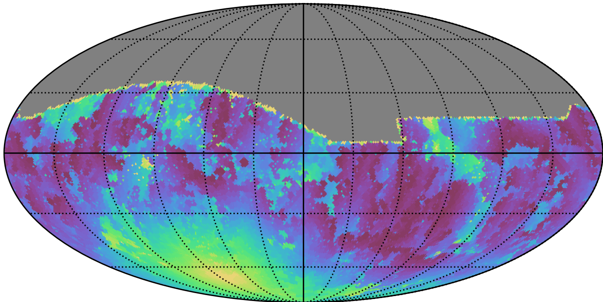
extra_ss_neo7_v3.4_10yrs All sky g band: Min moonDistance
