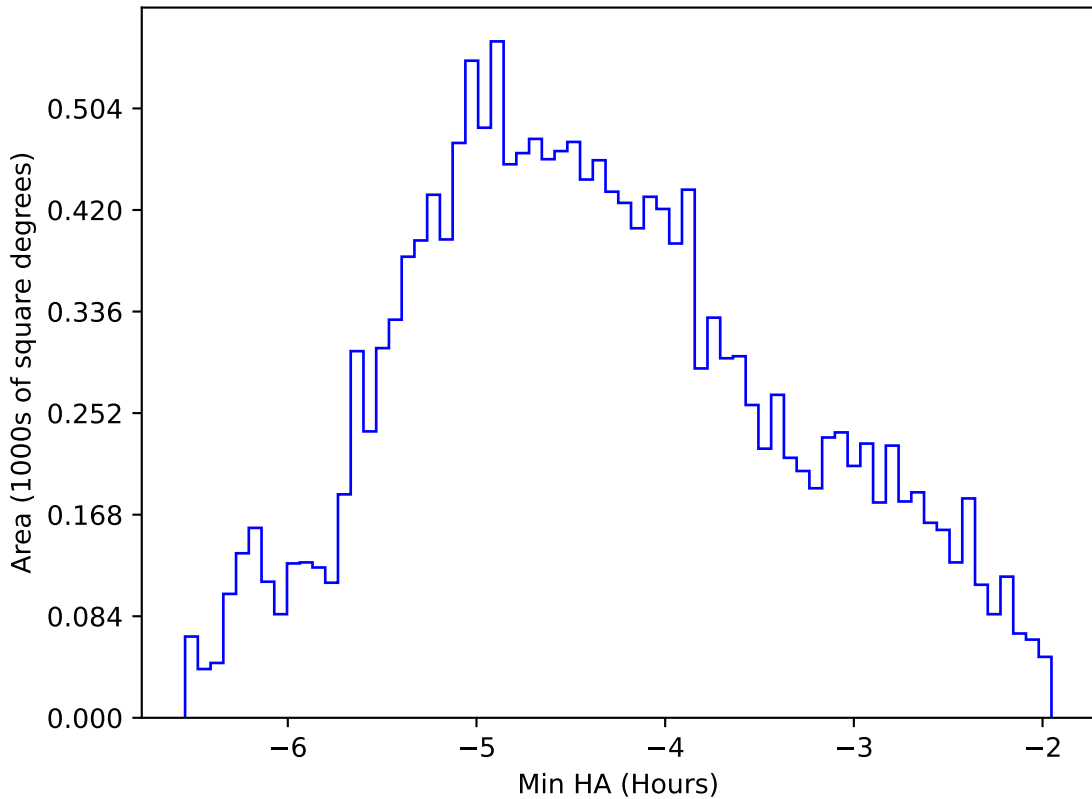
extra_ss_neo7_v3.4_10yrs WFD z band: Min HA
