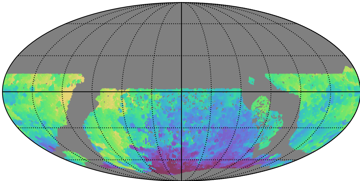
extra_ss_neo7_v3.4_10yrs WFD y band: Min HA
