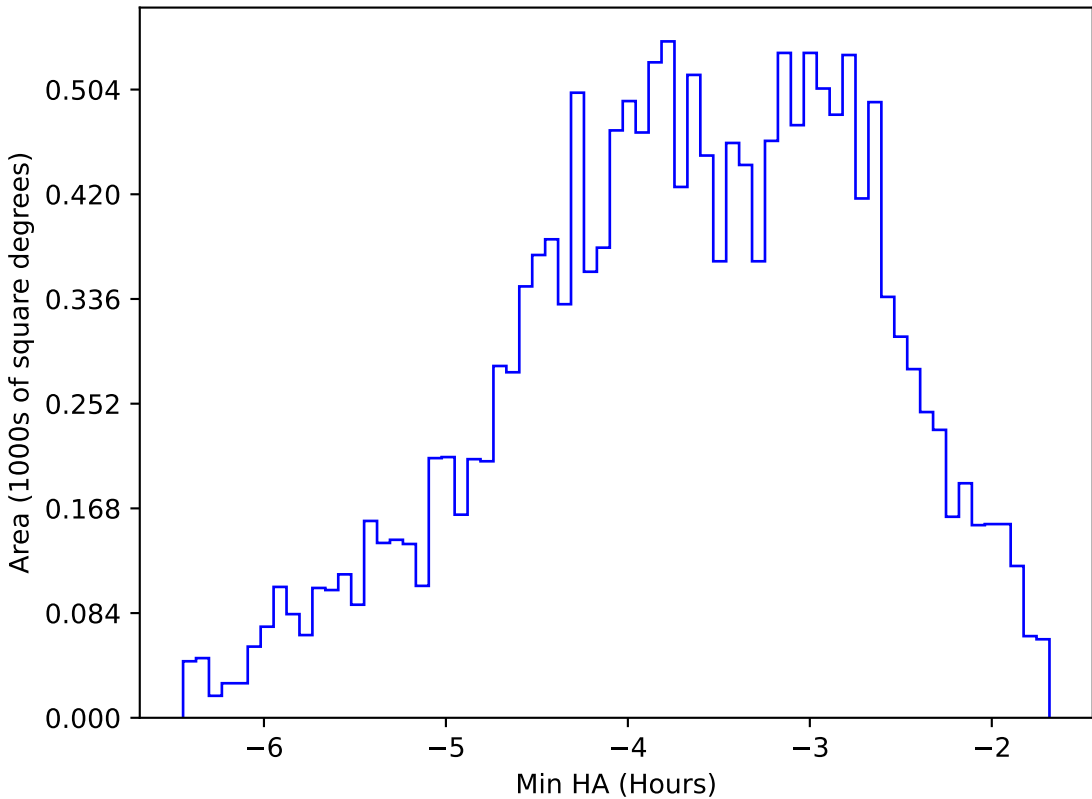
extra_ss_neo7_v3.4_10yrs WFD y band: Min HA
