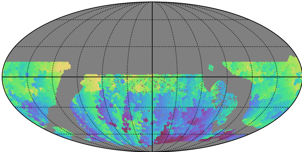
extra_ss_neo7_v3.4_10yrs WFD u band: Min HA
