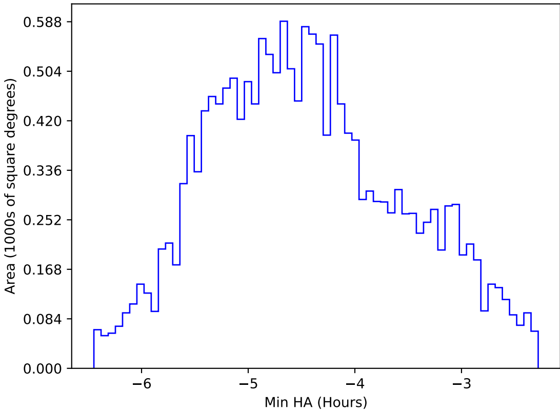
extra_ss_neo7_v3.4_10yrs WFD r band: Min HA
