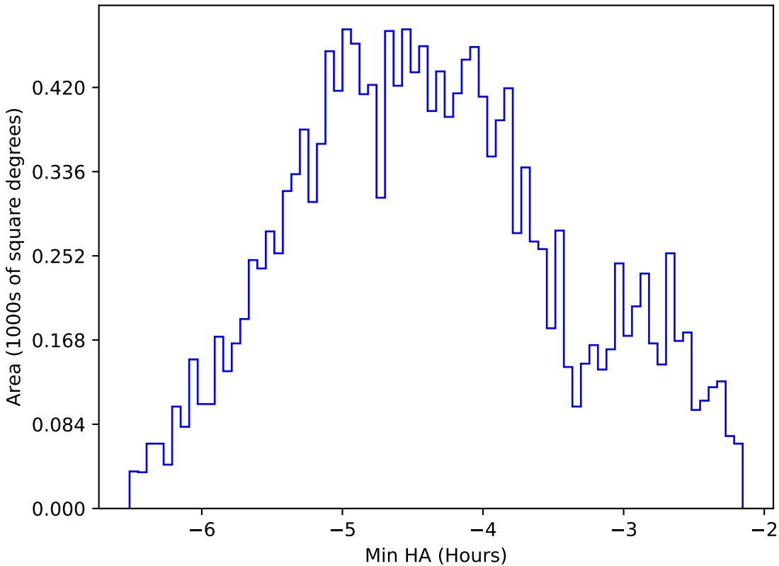
extra_ss_neo7_v3.4_10yrs WFD i band: Min HA
