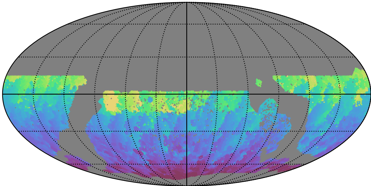
extra_ss_neo7_v3.4_10yrs WFD g band: Min HA
