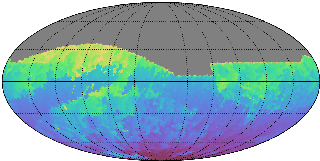
extra_ss_neo7_v3.4_10yrs All sky z band: Min HA
