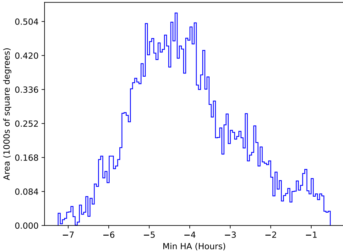
extra_ss_neo7_v3.4_10yrs All sky z band: Min HA
