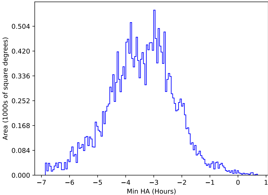
extra_ss_neo7_v3.4_10yrs All sky y band: Min HA
