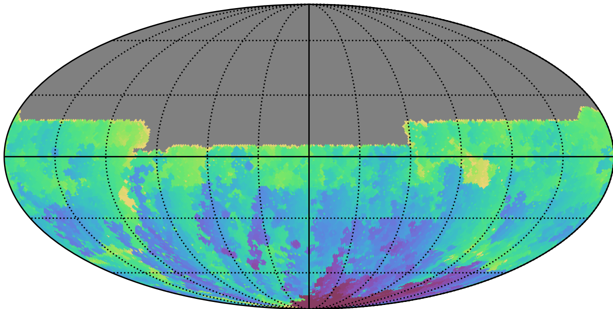
extra_ss_neo7_v3.4_10yrs All sky u band: Min HA
