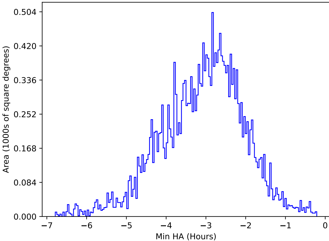
extra_ss_neo7_v3.4_10yrs All sky u band: Min HA
