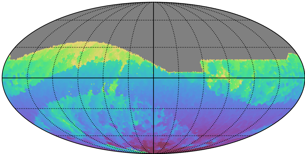
extra_ss_neo7_v3.4_10yrs All sky r band: Min HA
