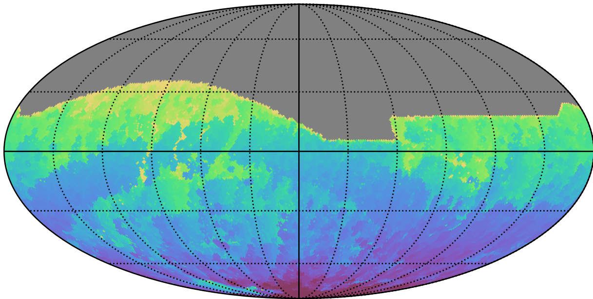
extra_ss_neo7_v3.4_10yrs All sky i band: Min HA
