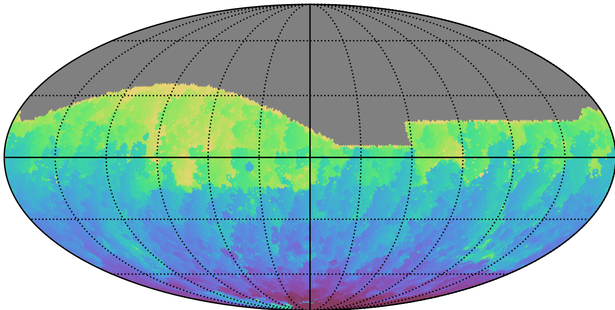
extra_ss_neo7_v3.4_10yrs All sky g band: Min HA
