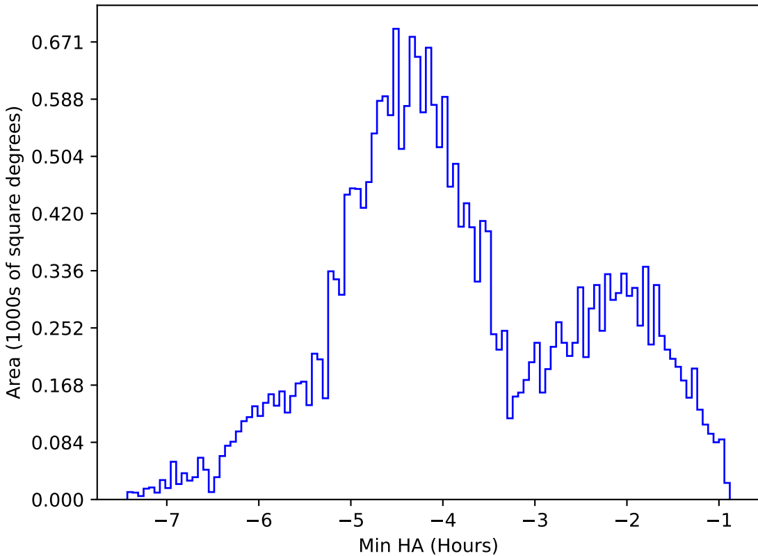
extra_ss_neo7_v3.4_10yrs All sky g band: Min HA
