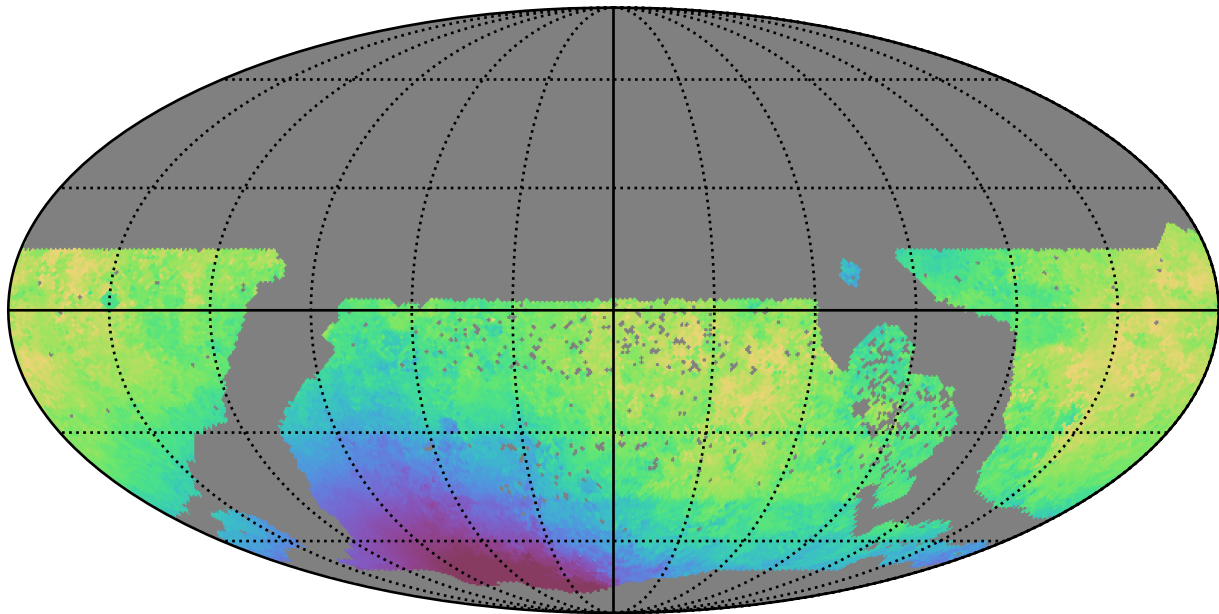
extra_ss_neo7_v3.4_10yrs WFD y band: Median solarElong
